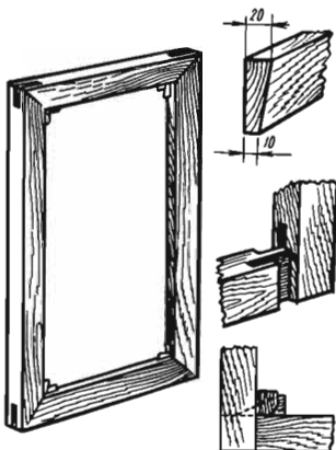
Рис. 107. Конструкция подрамника
