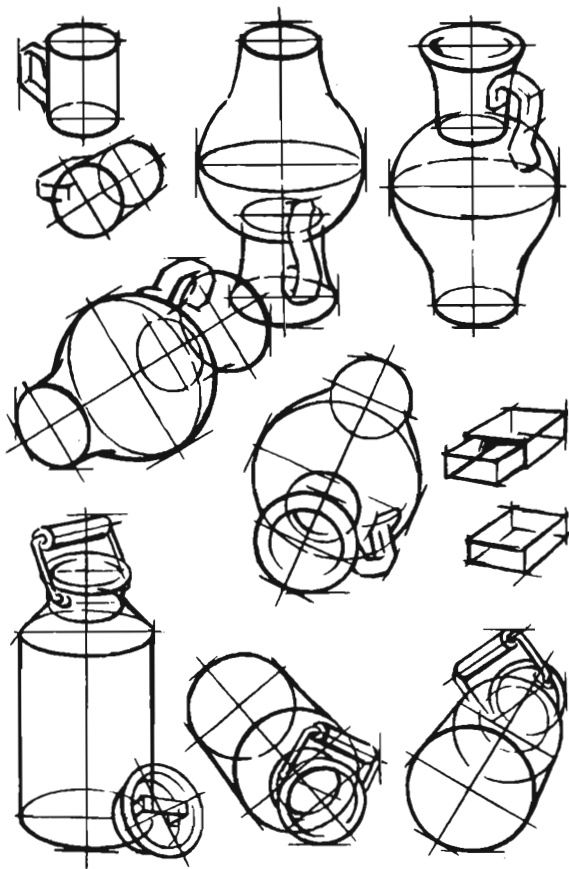
Рис. 48. Построение простых предметов обихода в ракурсе
