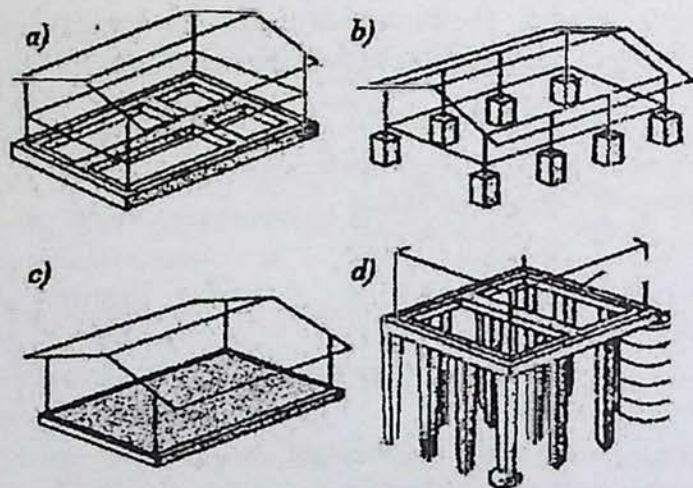
Poydevorlarning konstruktiv turlari:
