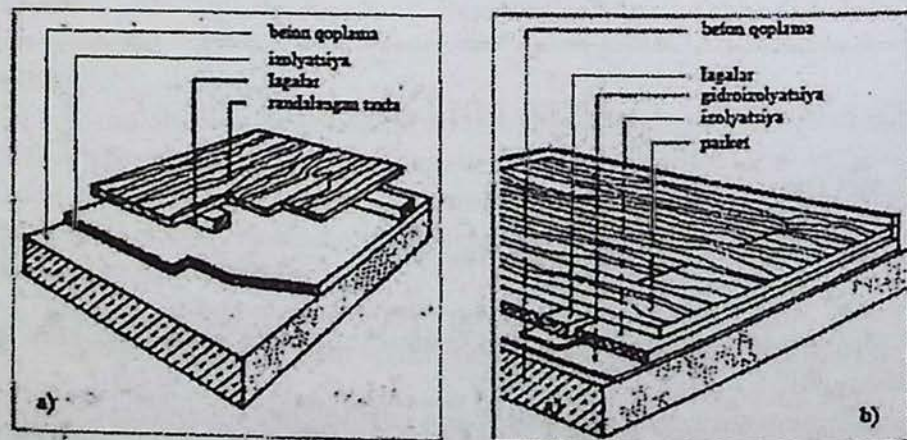
Pol konstruksiyasi:
