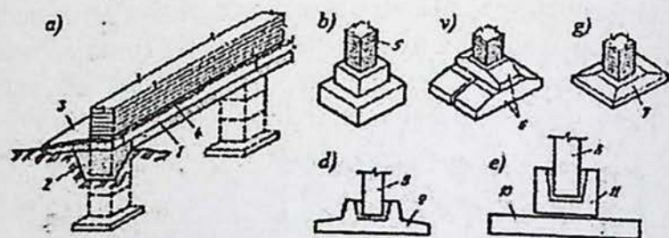
Ustunsimon poydevorlar:
