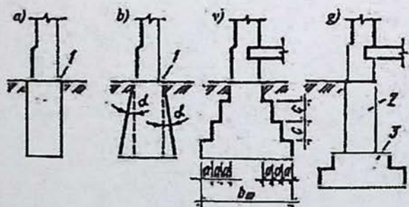
Lentasimon poydevorlarning ko'rinishi va tuzilishi:
