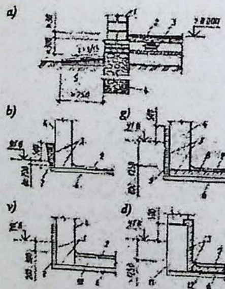
Kam qavatli hinolar elementlarini namlikdan himoyalash:
