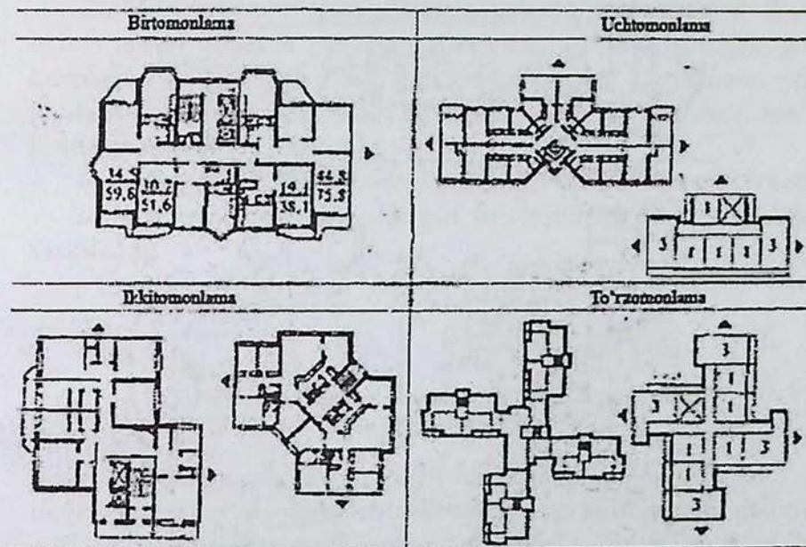
Ko'p seksiyali turarjoy uylarida seksiyalarni blokirovka qilish usullari
