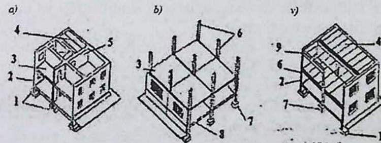
Sinchli binolarning konstruktiv sxemalari:
