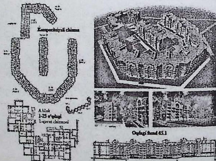
Blokirnyka qilingan seksiyalardan iborat turarjoy majmuasi loyihasi: — universal (cheklanmagan) mo'ljalli; — qisman cheklangan mo'ljalli (kenglikli); — cheklangan mo'ljalli (meridional).
