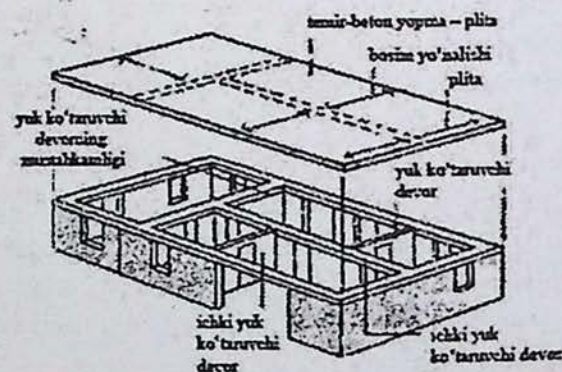
Temir-beton orayopmalar
