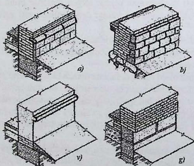
Sokol konstruksiyasi:
