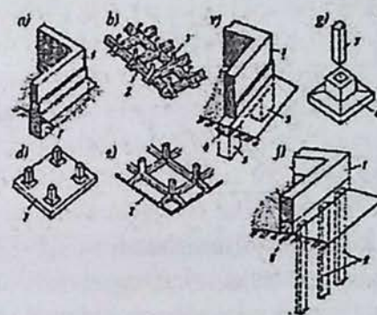
Poydevorlarning konstruktiv sxemalari:
