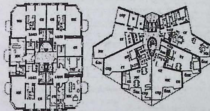
Minora turidagi bir seksiyali turarjoy binolari qavatlarining rejaları
