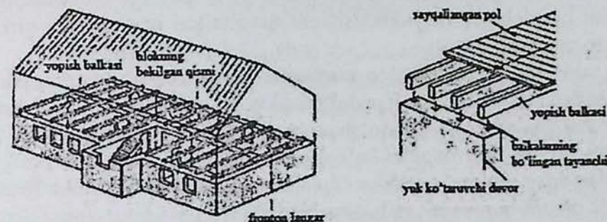
To'sinli yopma
