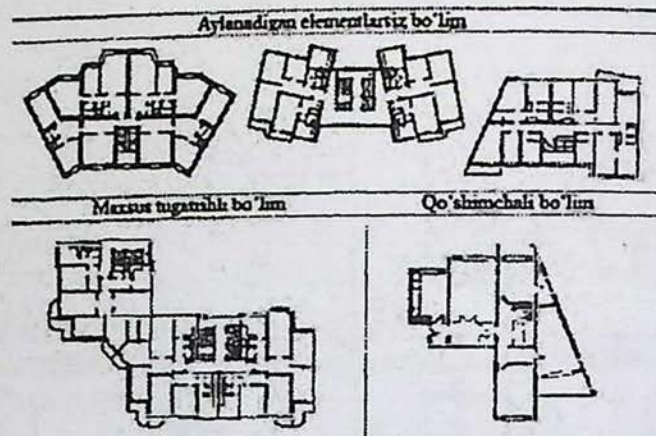
Ko'p seksiyali turarjoy uylarida burilish burchaklarini shakllantirish usullari
