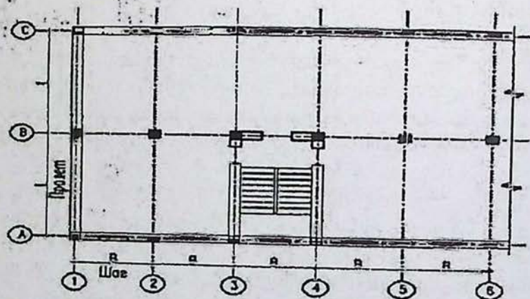
Loyihalashda modul tizimi va bino rejasida o'qlarning joylashishi
