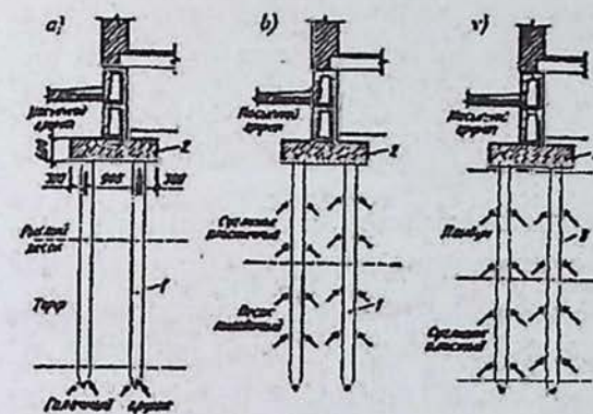
Qoziqoyoq poydevorlar:
