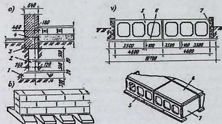
Yengillashtirilgan lentasimon yig'ma poydevorlarning konstruktiv yechimlari:
