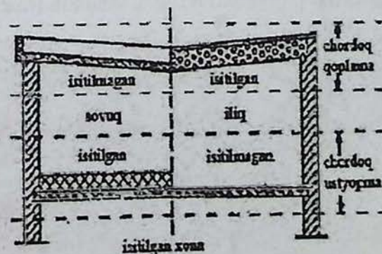
Chordoqli tom
