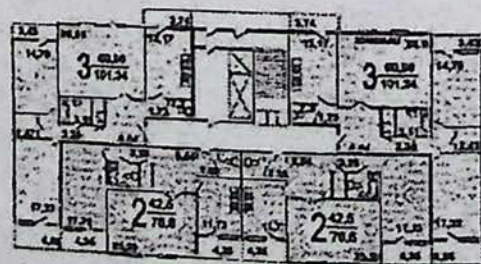
Turarjoyning oddiy seksiyasi rejasi
