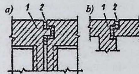
Deformatsiya choklari:
