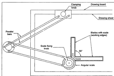
Figure 1.2 Mini drafter
