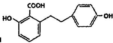
Lunular kislotasi
