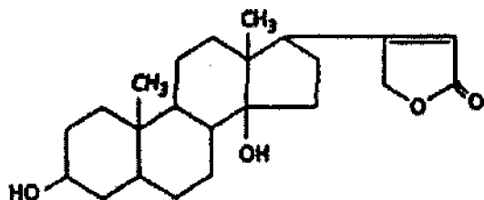
Digitoksigenin
