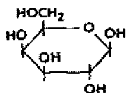
\beta -D-galaktoza
