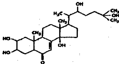
\alpha - Ekdizon
