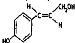
Para-kumar spirti
