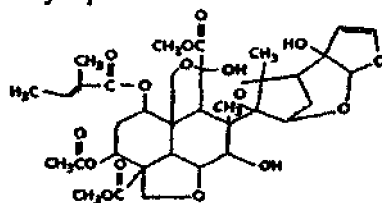
Azadiraxtin
