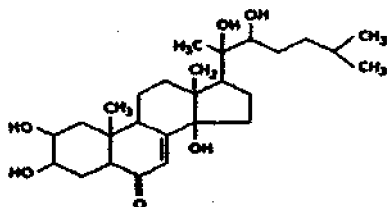
Ponasteron A
