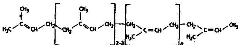
Kauchukning formulasi.
