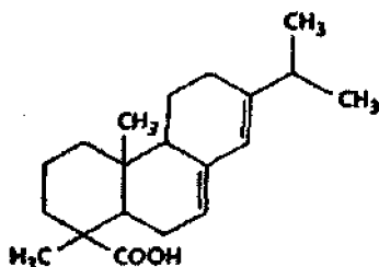
Abiet kislotasi
