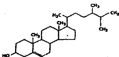
Sitosterol
