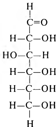
Glukoza
