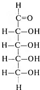
Riboza
