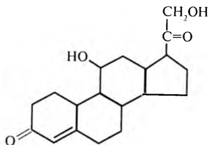
Kortikosteron
