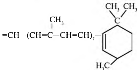
\beta -karotin
