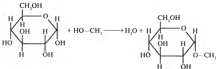
Glukoza
