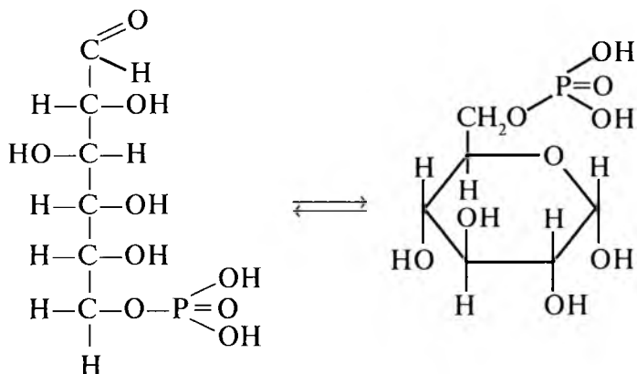
Glukoza-6-fosfat
