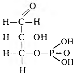
Fosfoglitserin aldegidi
