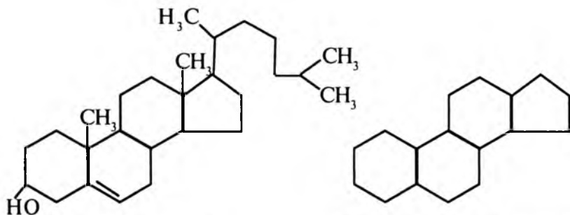
Xolesterin
