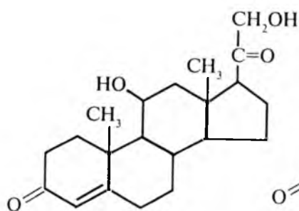
Gidrokortizon
