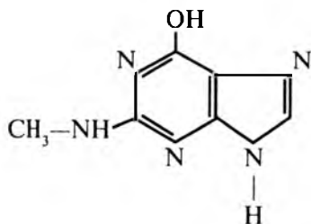
N 2 -metilguanin
