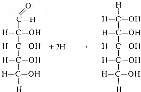
Riboza
