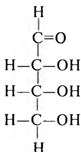
Eritroza
