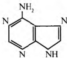
adenin
