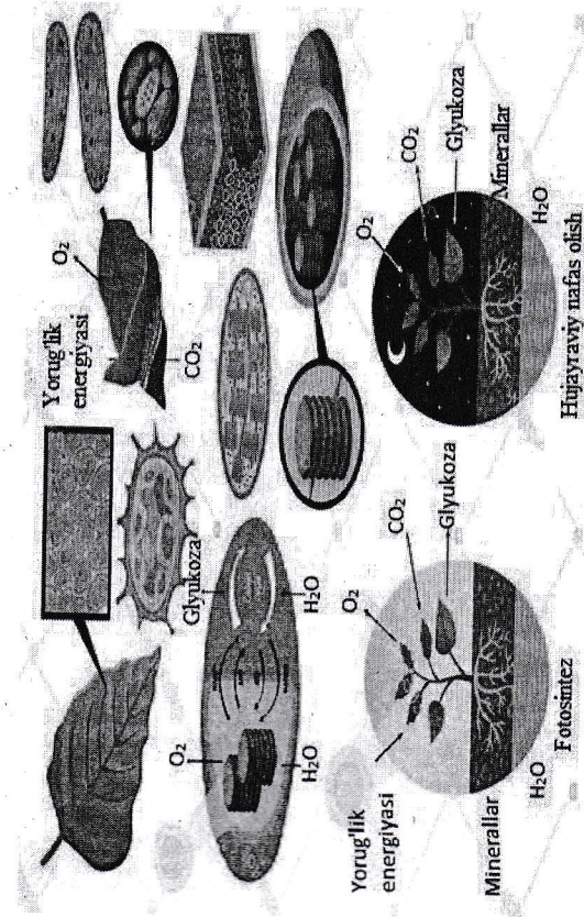
14-rasm. Fotosintez jarayoni.
