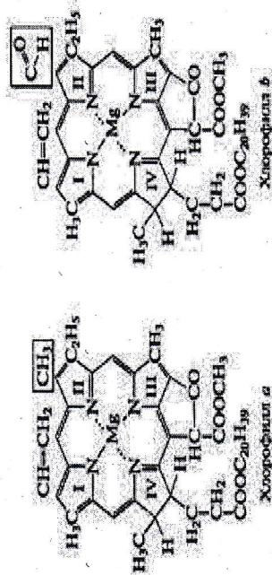
15- rasm. Xlorofill "a" va xlorofill "b" ning tuzilmaviy formulasi.
