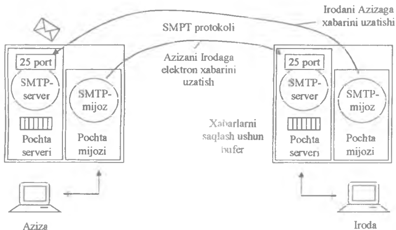
11.1-rasm. Mijoz va serverning bevosita muloqot sxemasi.
