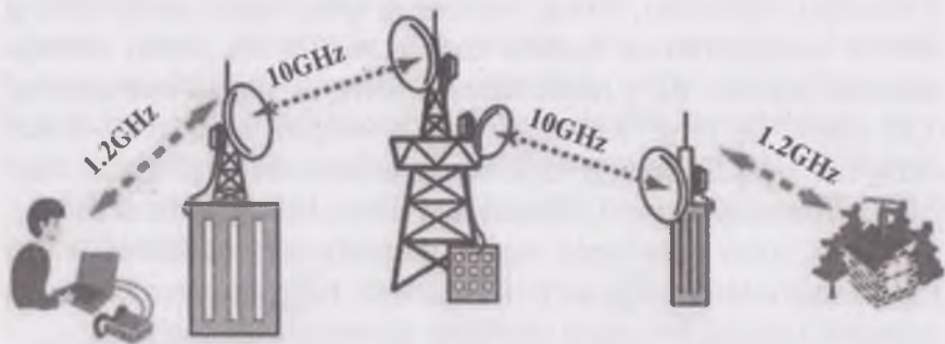
1.9.5-rasm. Mikroto'liqinli aloqa
