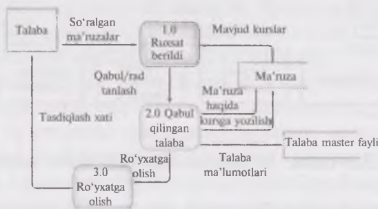
2.3.5-rasm. Maʼlumotlar oqimi diagrammasi
