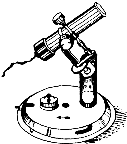
17-rasm. Termoelektrik aktinometrning tashqi ko‘rinishi.
