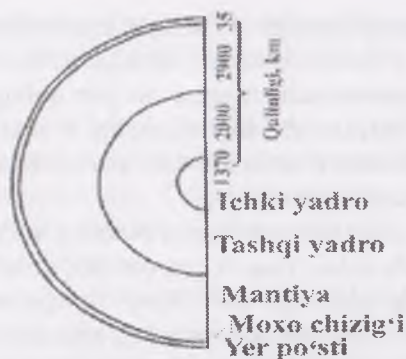
4.2-rasm. Yerning ichki tuzilishi'
