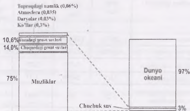
9.1-rasm. Gidrosferada suvning miqdori 1
