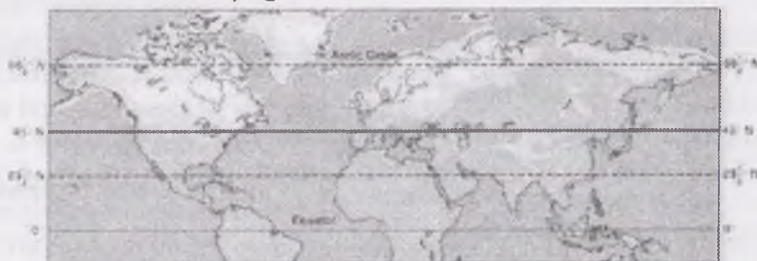
12.5-rasm. Pleystotsen davri materik muzliklari
