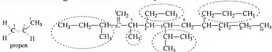
2-ikkilamchibutil-3-metil-5-izopropil-7-propil-4-etildetsen-1
