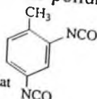
toluol-2,6-diizotsianat
