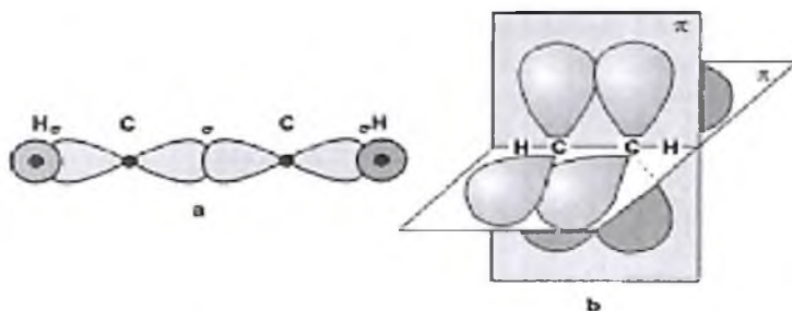
5-rasm. Atsetilen molekulasida kimyoviy bog'larning hosil bo'lishi: a) \sigma - bog'lar; b) \pi - bog'lar.
