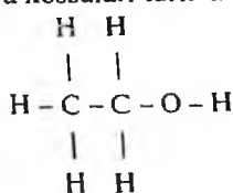
etil spirti
