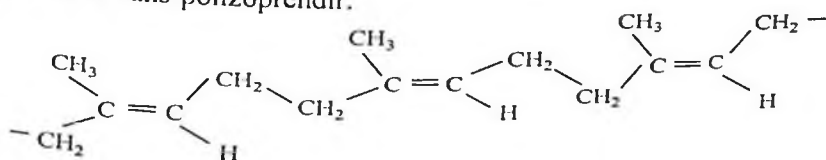
trans-polizopren
