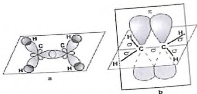
4- rasm. Etilen molekulasida kimyoviy bog'larning hosil bo'lishi: a) \sigma - bog'lar; b) \pi - bog'lar
