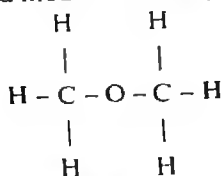
dimetil efir
