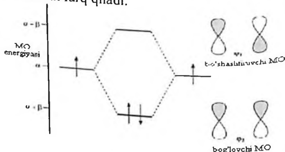
Etilen molekulasida \pi -bog'ning hosil bo'lishi
