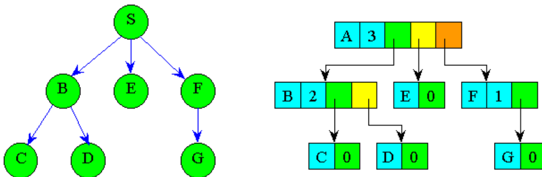
4.5-rasm. Daraxtni grafik shakldagi va uning chiziqsiz ro'yxat shaklidagi ifodalanishi
