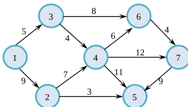
4.24-rasm. Yo‘naltirilgan va vaznga ega graf
