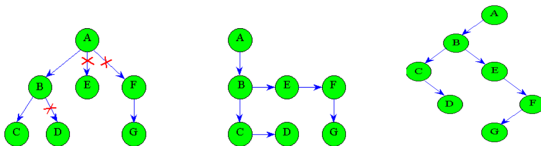
4.8-rasm. m-o‘lchovli daraxtni binar ko‘rinishga keltirish
