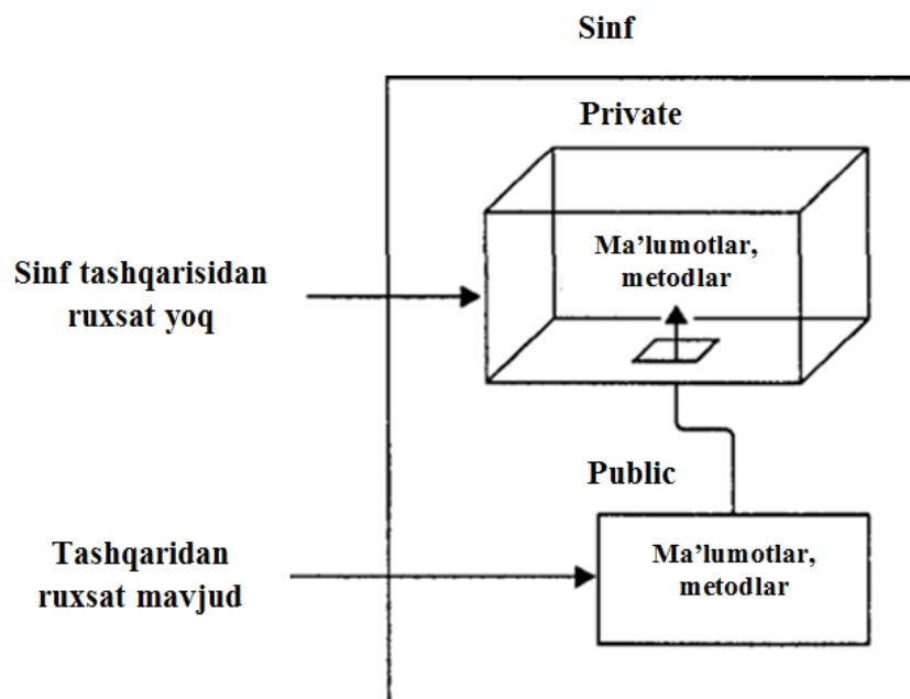
1.5-rasm. Sinf a’zolariga murojaatni amalga oshirish sxemasi
