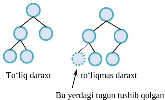
4.13-rasm. Heap treeni to'g'ri va noto'g'ri tashkil etilganligi
