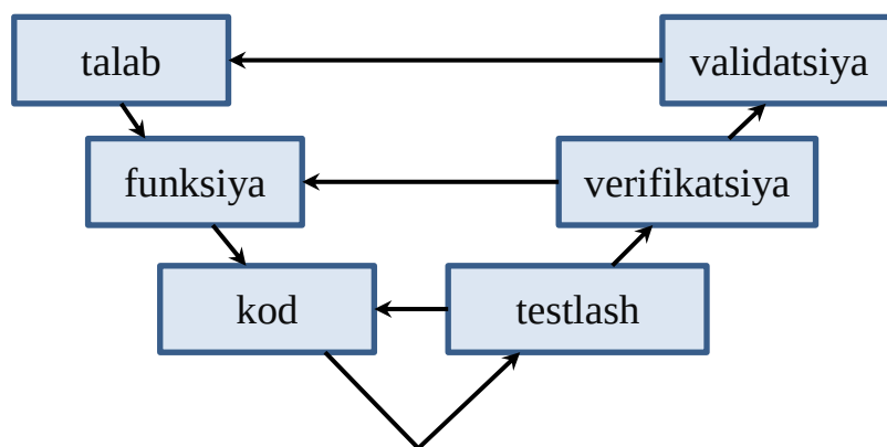
5.1-rasm. Testlash, verifikatsiya va validatsiya
