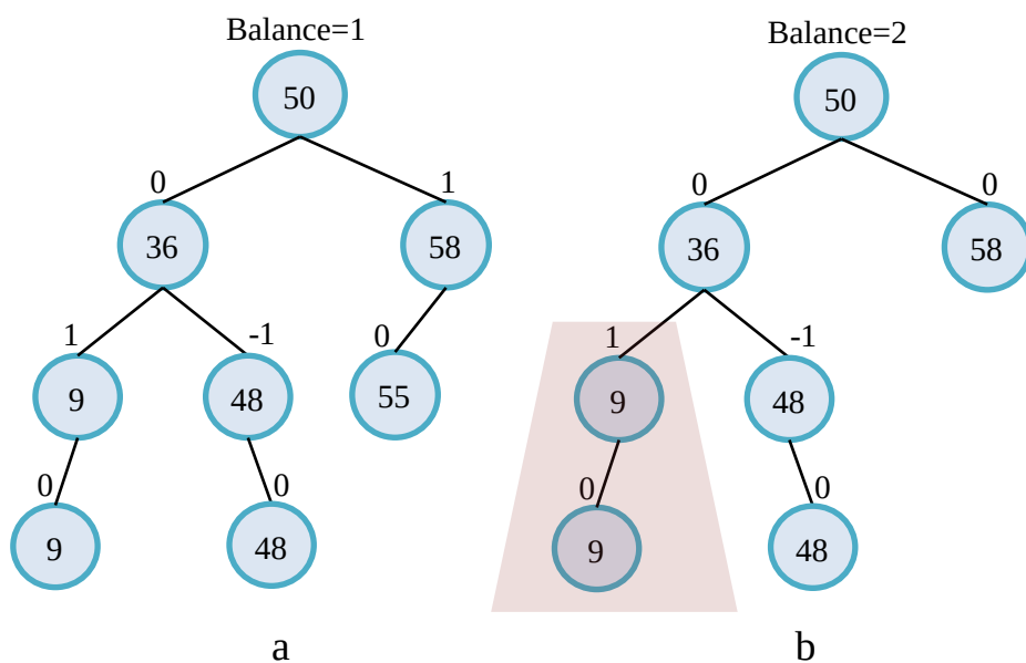
4.22-rasm. Tugunlar muvozanatlanganlik darajasi; a-AVL daraxt, b-AVL daraxt emas
