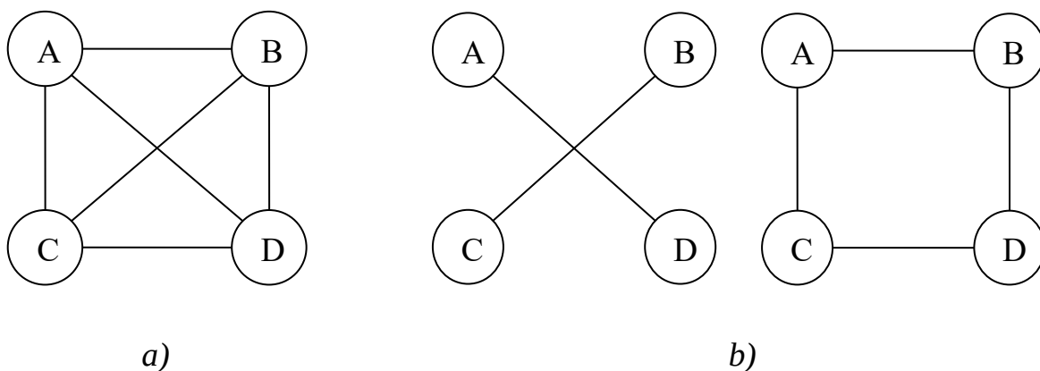
4.27-rasm.a) to'liq graf b) graf va uning to'ldiruvchisi
