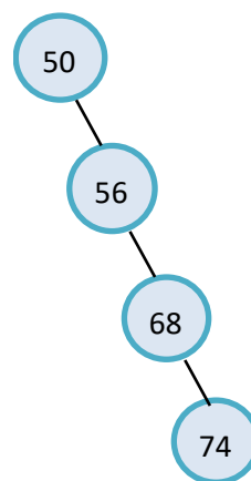
4.20-rasm. O‘rish tartibida kelib tushgan elementlardan hosil qilingan binar qidiruv daraxti
