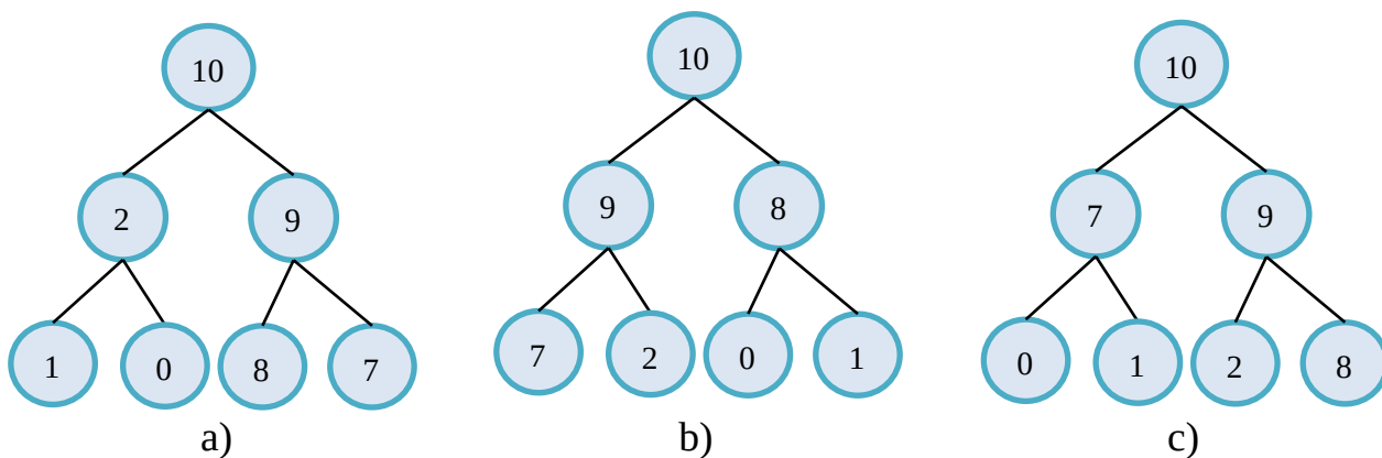
4.12 – rasm. Bir xil sonlardan tashkil topgan heap tree tuzilmalari
