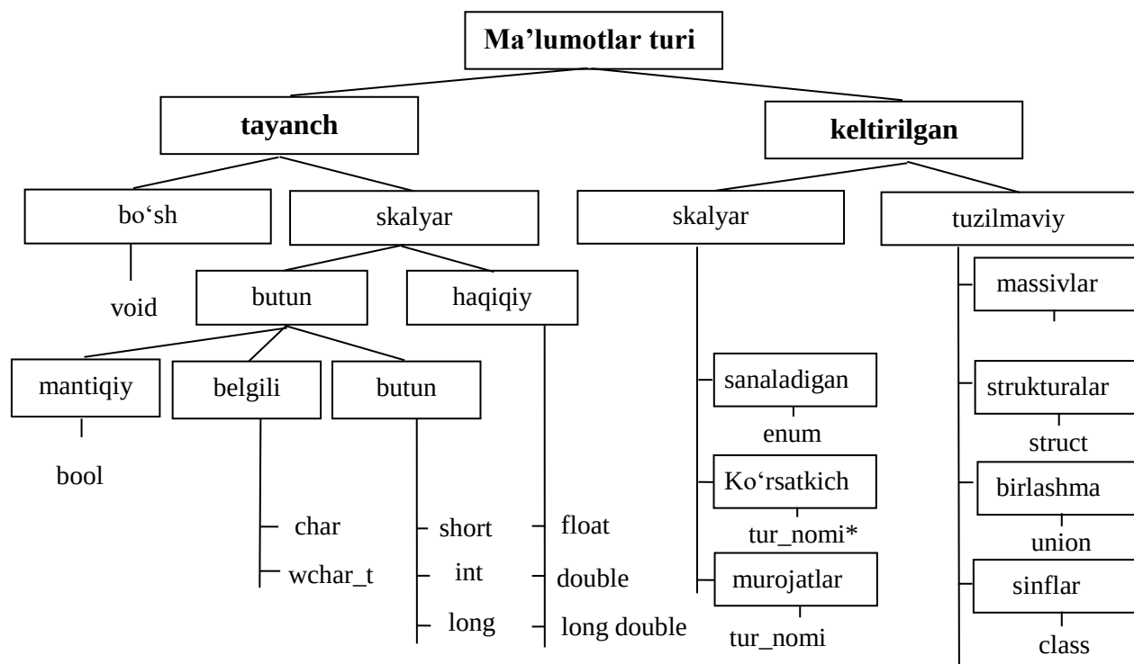
1.3-rasm. Ma'lumotlar turlarining sinflanishi
