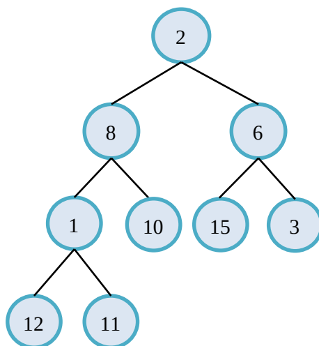
4.10-rasm. Massivdan daraxt hosil qilish
