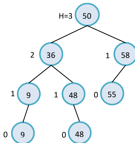
4.21-rasm. Binar qidiruv daraxti tugunlari balandliklari
