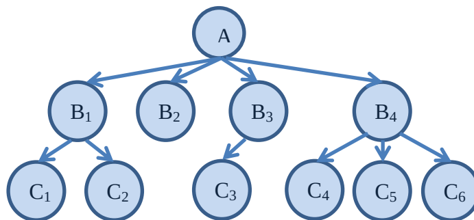
5.3-rasm. Ierarxik ma'lumotlar modeli tuzilishi
