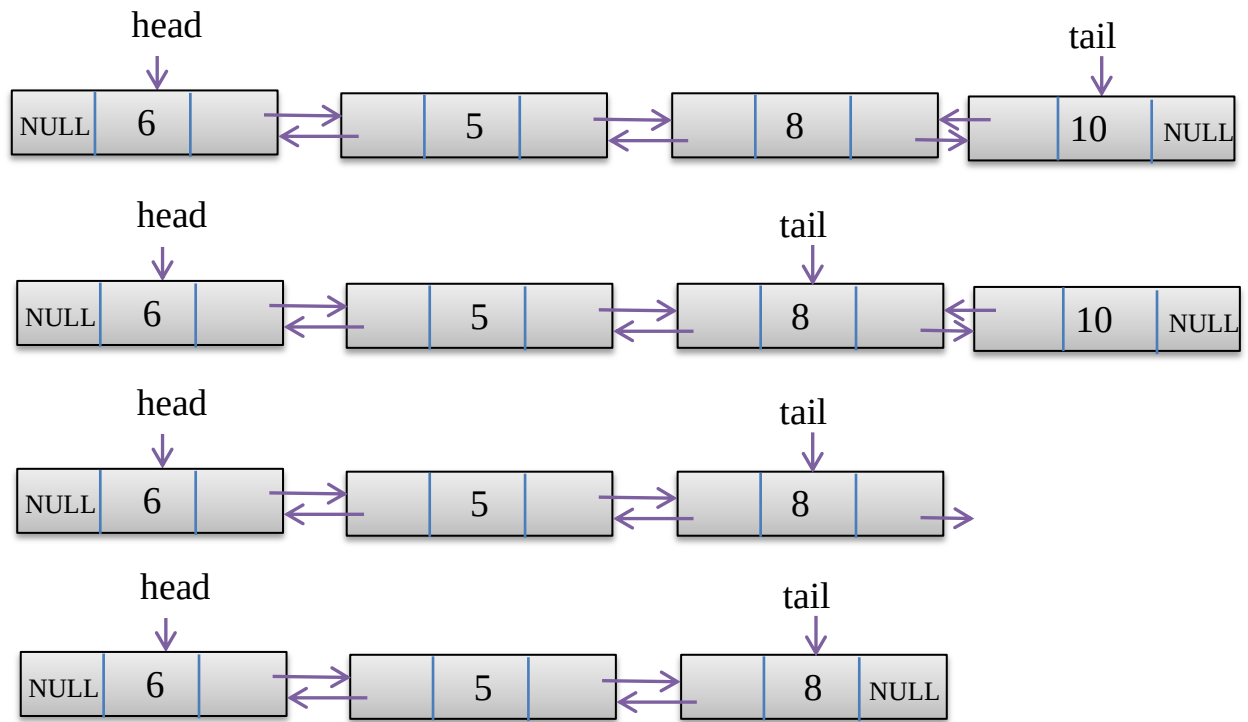
3.3-rasm. Ikki bog‘lamli ro‘yxat oxiridan elementni o‘chirish amali
