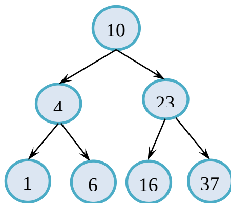
4.7-rasm. Binar qidiruv daraxti
