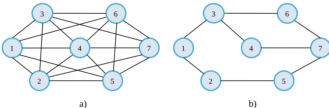
4.28-rasm.a) to'yingan graf ( D=0.76 ) b) siyrak graf ( D=0.38 )
