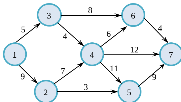
4.29-rasm. Vaznga ega bo‘lgan yo‘naltirilgan graf
