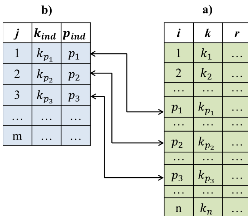
2.1-rasm. a) asosiy ma'lumotlar jadvali; b) indekslar jadvali
