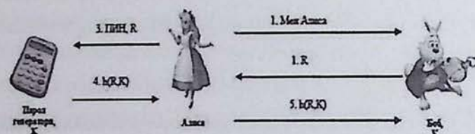
3.3-rasm. Tokenga asoslangan autentifikatsiya jarayoni
