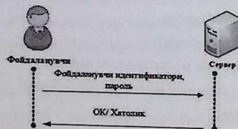
3.1-rasm. Parolga asoslangan mashina-insonni autentifikatsiyalash jarayoni
