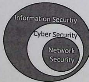
3.9-rasm. Kiberxavfsizlik.
