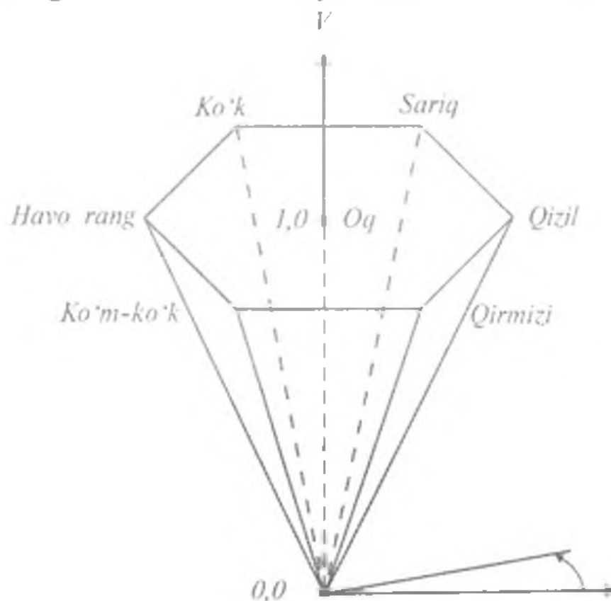
1.11-rasm. Ranglarni indeksli kodlash usuli
