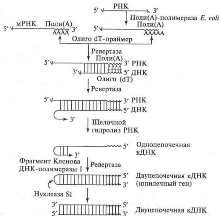
Рис. 178. Схема получения кДНК с использованием ревертазы вируса птичьего миелобластома и трех дополнительных ферментов: поли(А)-полимеразы, фрагмента Кленова ДНК-полимеразы I и нуклеазы S1 (разрушает характерную шпильку в молекуле кДНК, которую образует ревертаза)
