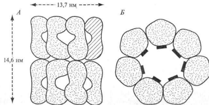
Рис. 21. Структура шаперонинового комплекса GroEL:
