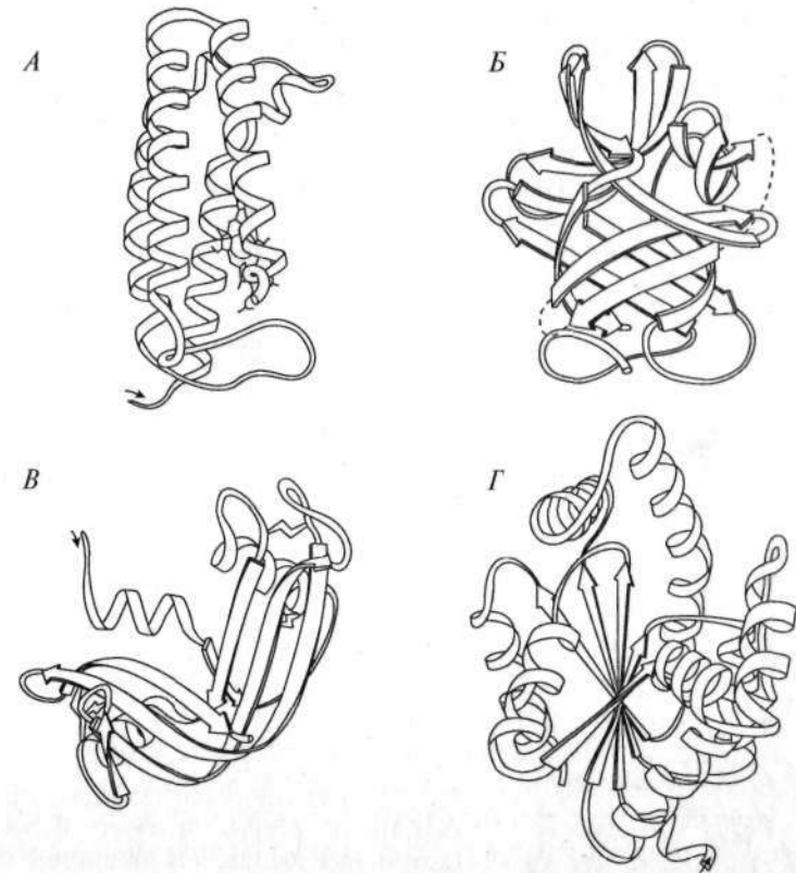
Рис. 11. Белки, относящиеся к различным структурным группам в зависимости от представительства элементов вторичной структуры:
