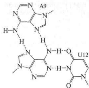
Рис. 53. Образование А·U·А-триплета в тРНК
