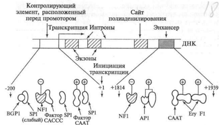
Рис. 133. Присоединение белков, усиливающих (+) и ослабляющих (-) транскрипцию, к регуляторным элементам гена \beta -глобина курицы (пояснения в тексте) (по Б.Албертсу и др., 1994)
