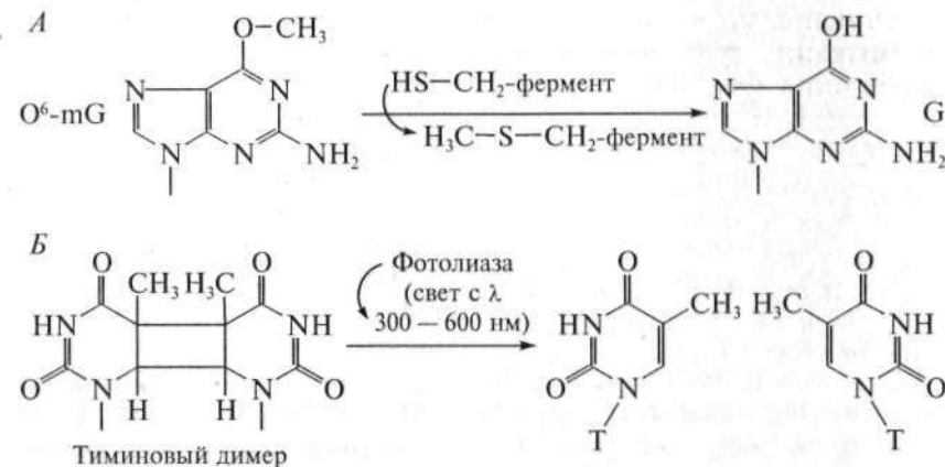
Рис. 170. Примеры прямой репарации повреждений в ДНК:
