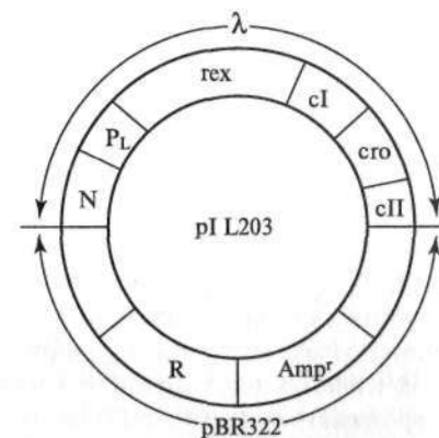
Рис. 183. Упрощенная схема строения плазмидного вектора pI L203: N, rex, cro, cI, cII — гены фага \lambda ; P_L — регулируемый промотор; Amp^r — ген устойчивости к ампициллину
