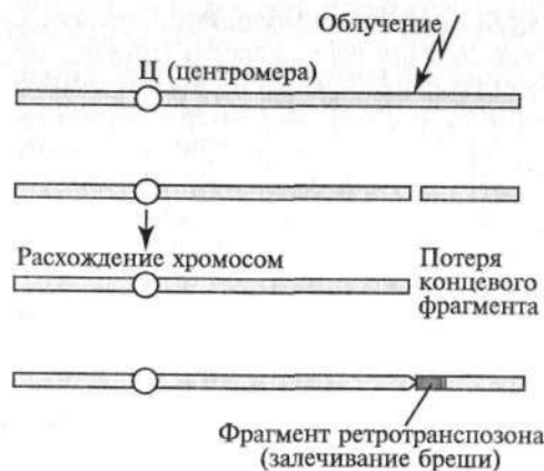
Рис. 99. Устранение двунитевого разрыва ДНК с помощью ретротранспозона
