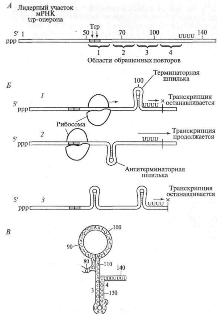
Рис. 125. Схема регуляции транскрипции мРНК trp-оперона с участием рибосомы:
