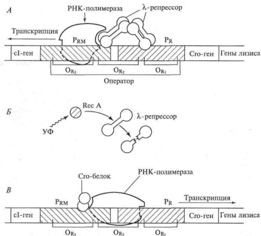
Рис. 128. Схема взаимодействия молекул \lambda -репрессора и Сго-белка с зоной оператора ДНК фага \lambda :
