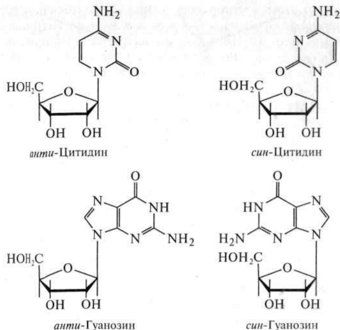
Рис. 40. Анти- и син-конформации в нуклеотидах
