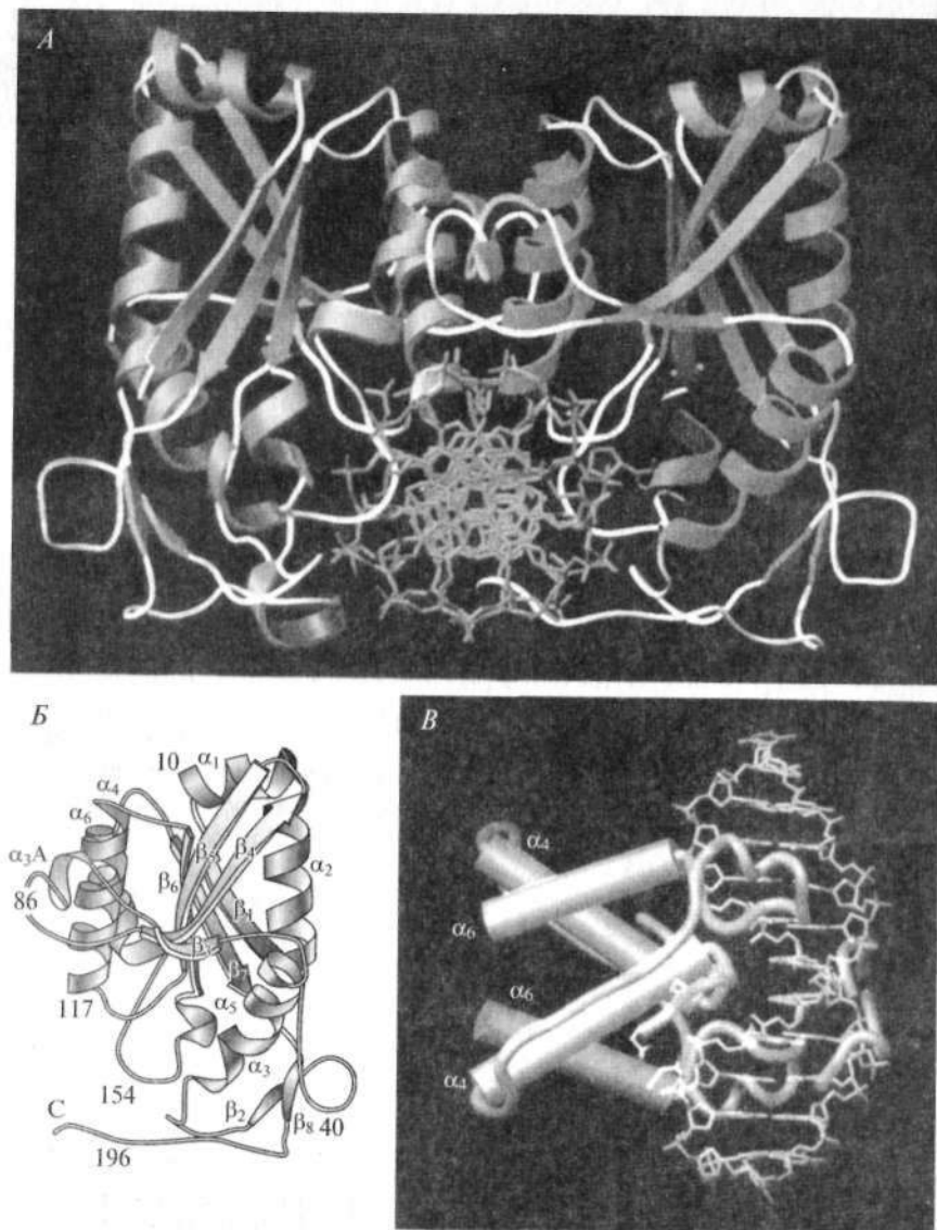
Рис. 27. Структура рестриктазы Bam HI, взаимодействующей с ДНК: А — структура комплекса Bam HI-ДНК. Две субъединицы фермента (L и R) расположены соответственно слева и справа от обозначенной внизу молекулы ДНК; Б — R-субъединица рестриктазы Bam HI (показано расположение \alpha -спиралей ( \alpha_1 — \alpha_6 ) и \beta -слоев ( \beta_1 — \beta_8 ); цифрами обозначено расположение отдельных аминокислотных остатков начиная с N-конца молекулы, С — карбоксильный конец молекулы); В — взаимодействие отдельных структурных элементов R- и L-субъединиц рестриктазы с молекулой ДНК (спирали и петли вторичной структуры субъединицы R выделены темным цветом, соответствующие элементы L-субъединицы — серым)
