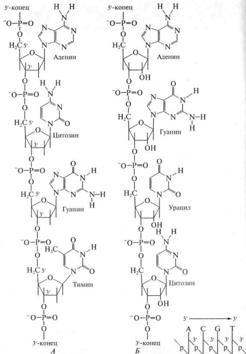
Рис. 35. Связь между нуклеотидами в полинуклеотидной цепи:
