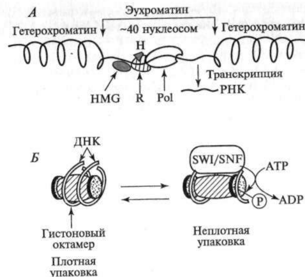
Рис. 138. Деконденсация хроматина в зоне активной транскрипции:
