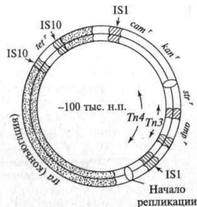
Рис. 72. Структура типичной конъюгативной R-плазмиды.
