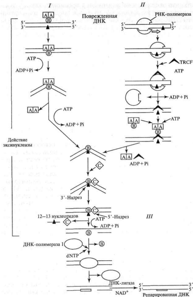
Рис. 172. Схема нуклеотидной эксцизионной репарации у E. coli с участием эксинуклеазы:
