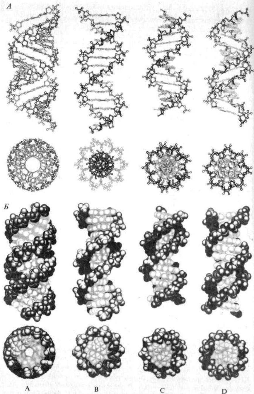
Рис. 44. А-, В-, С- и D-формы ДНК (вид сбоку и сверху) (В. Зенгер, 1987): А — скелетная модель; В — объемная модель
