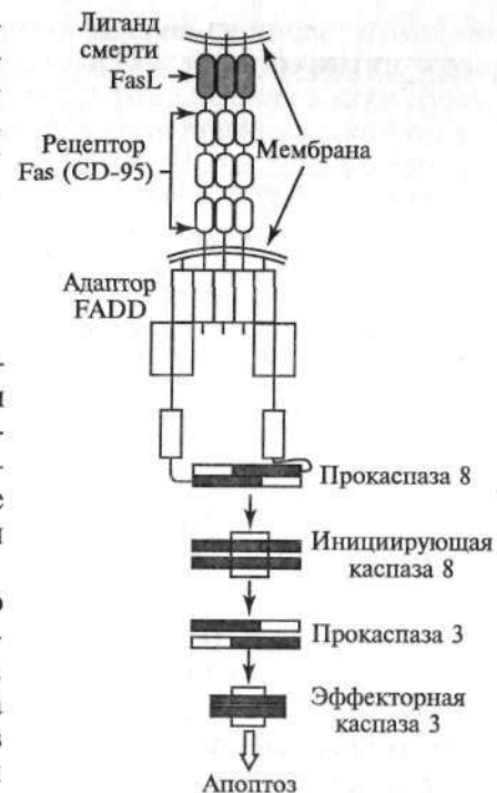
Рис. 176. Каскадная система индукции апоптоза, включающая функционирование лиганда FasL, рецептора CD-95, адаптора FADD, инициаторной каспазы 8 и эффекторной каспазы 3
