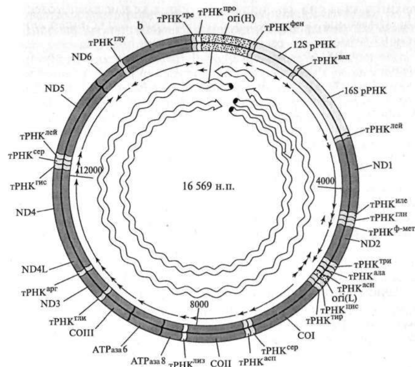
Рис. 103. Митохондриальная ДНК человека.
