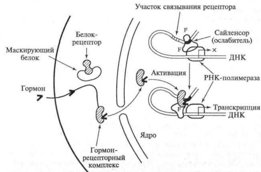
Рис. 134. Воздействие стероидных гормонов на транскрипцию (по В.А.Гвоздеву, 1996):
