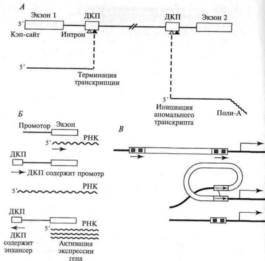
Рис. 96. Эффекты внедрения ретротранспозона внутрь гена или около гена: А — нарушение транскрипции при внедрении в интрон; Б — усиление экспрессии гена при внедрении в 5'-район гена; В — образование подвижного промотора в процессе гомологической рекомбинации после удаления тела элемента
