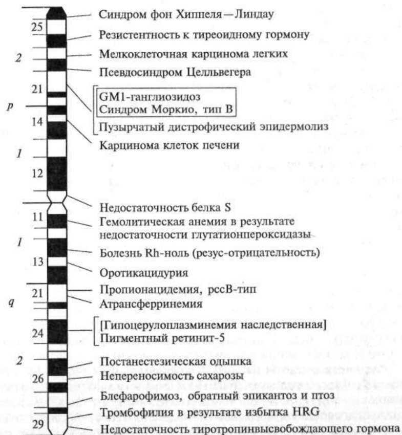
Рис. 100. Генетическая карта 3-й хромосомы человека
