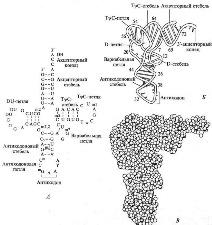
Рис. 55. Структура дрожжевой тРНК Р he :
