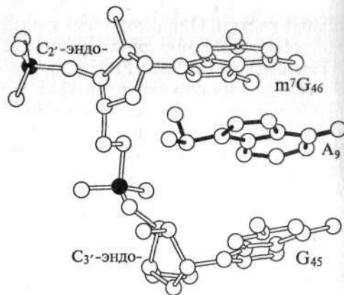
Рис. 54. Интеркаляция А 9 между остатками m 7 G 46 и G 45 в тРНК.
