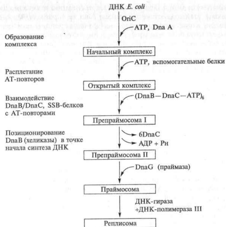
Рис. 110. Схема инициации репликации хромосомы E. coli
