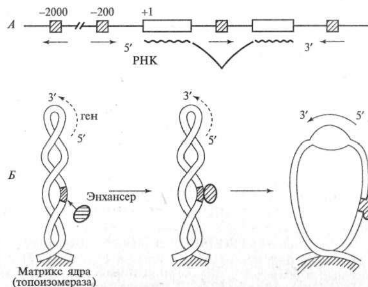
Рис. 82. Энхансеры эукариотических генов:
