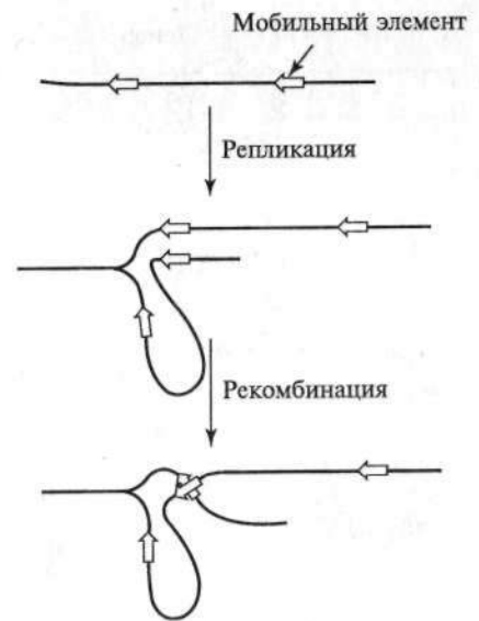
Рис. 76. Механизм образования дупликаций за счет гомологической рекомбинации по мобильным элементам (неравный кроссинговер)
