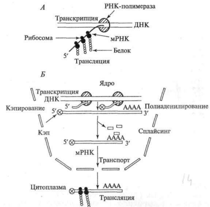
Рис. 121. Различия в транскрипции и трансляции у прокариот (А) и эукариот (Б).
