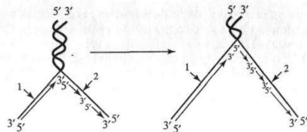
Рис. 105. Синтез цепей ДНК в репликативной вилке.
