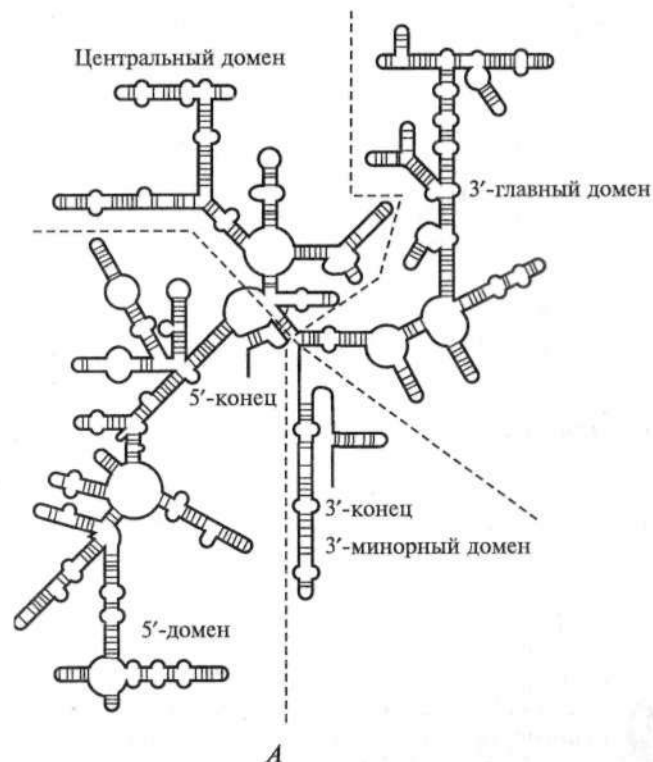
Рис. 56. Структуры 16S рРНК E. coli :
