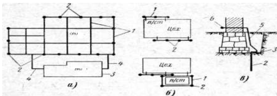
45- rasm. a) va b) - Ochiq va yopiq taqsimot qurilmalarni erga ulash sxemalari; 1- metall setkasi; 2- vertikal elektrod; 3-gorizontall yer ulagich;
