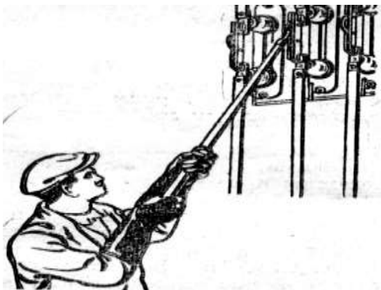
61- rasm. Tezkor himoyalovchi shtanga yordamida taqsimlash uskunalarida ayiruvchi pichoqlarni yoqish va o'chirish
