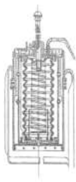
6-rasm. Universal gaz tahlil qilish qurilmasi UG-2.
