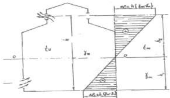
11-rasm. Tabiiy shamollatishda sanoat korxonasida hosil bo'ladigan bosimlarning taqsimlanish.
