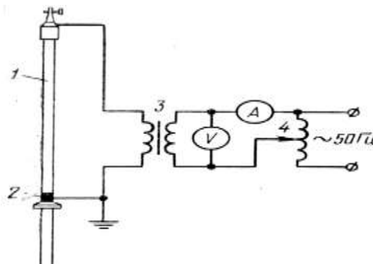
59-rasm. Shtangani sinovdan o’tkazish sxemasi.
