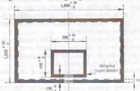
88-rasm. "Shchit" (savat ortidagi to'siq) o'lchamlari
