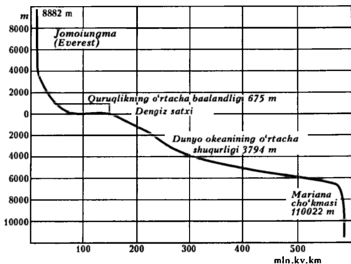
25-rasm. Gipsografik egri chiziqli.
