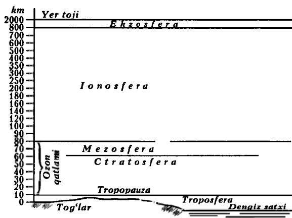
26-rasm. Atmosferaning tuzilishi.
