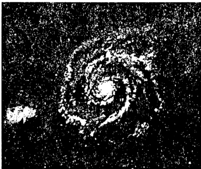
10-rasm. «Girdob» spiral tumanligi (L.P.Shubayev, 1975)
