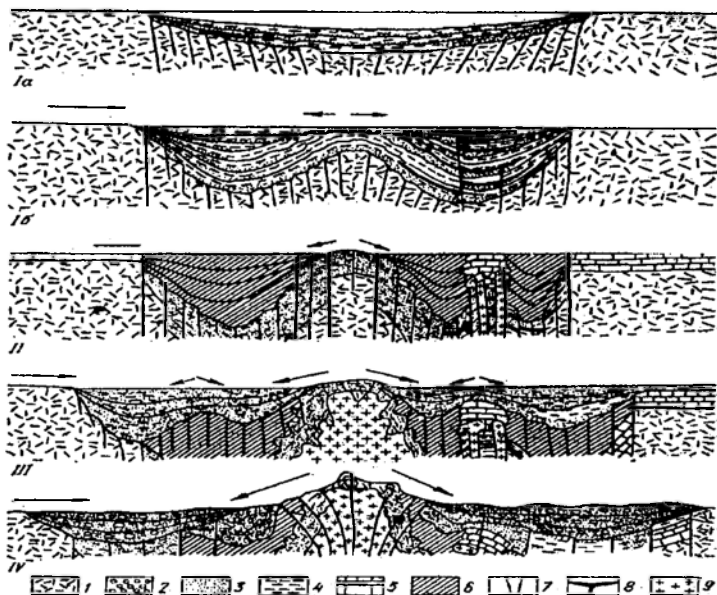
22-rasm. Geosinklinallarning rivojlanish bosqichlari (V. Ye. Xain bo'yicha)
