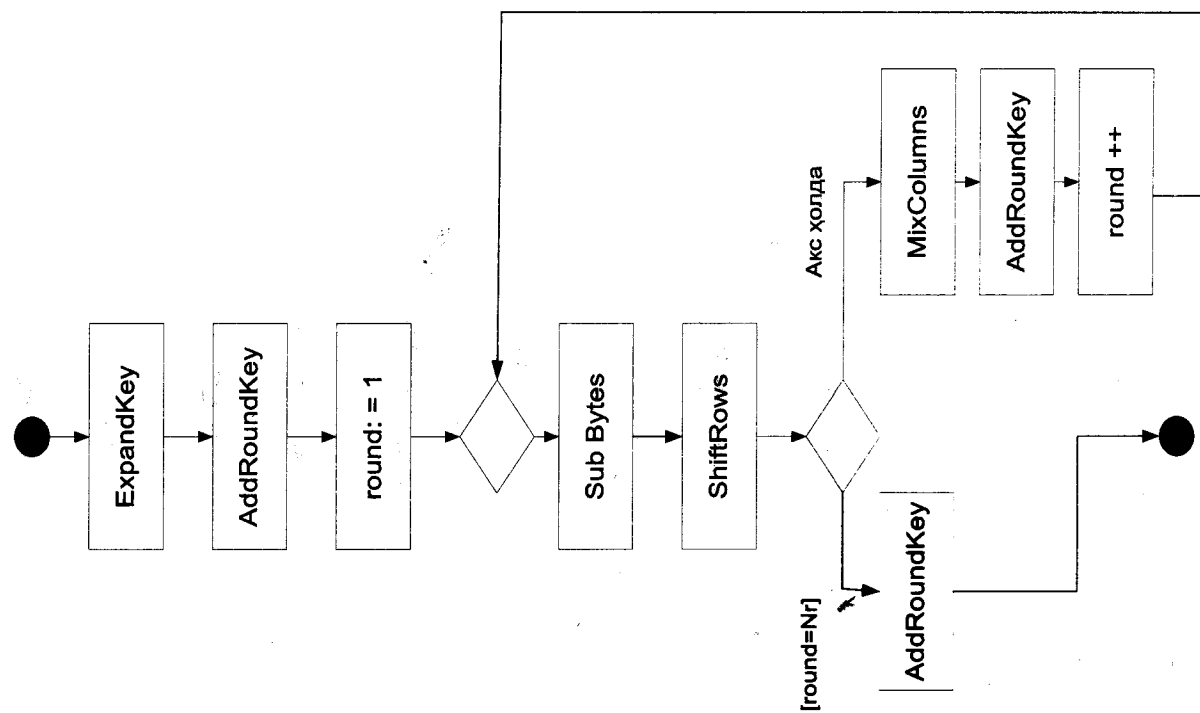
5.12-rasm. Shifrlash jarayoni.
