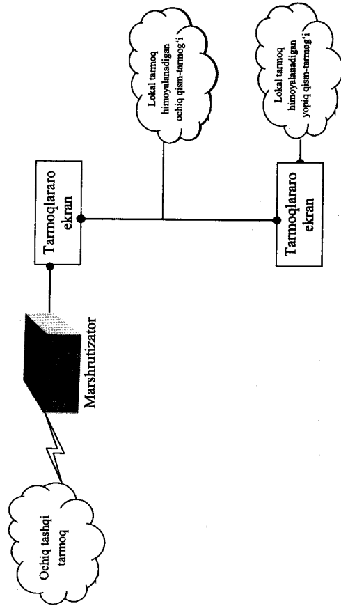
8.15-rasm. Ikki tarmoq interfeysli ikki tarmoq brandmauer asosida yopiq va ochiq qismtarmoqlarni alohida himoyalash sxemasi.
