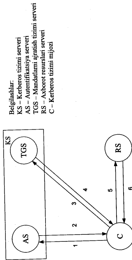
6.2-rasm. Kerberos protokolining ishlash sxemasi.
