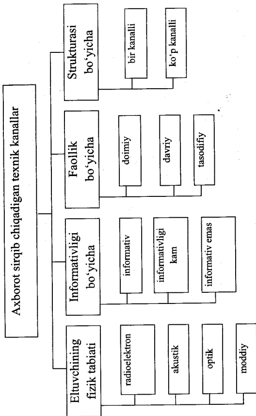
10.3-rasm. Axborot sirqib chiqadigan texnik kanallarning turkumlanishi.
